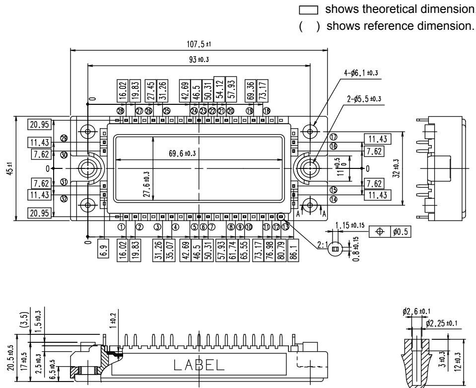
Section A-A
