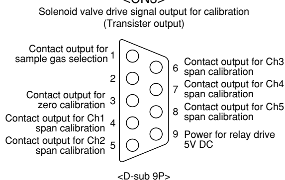
Connector <CN3>
