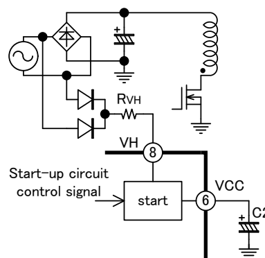
Fig.31 VH pin circuit (1)
