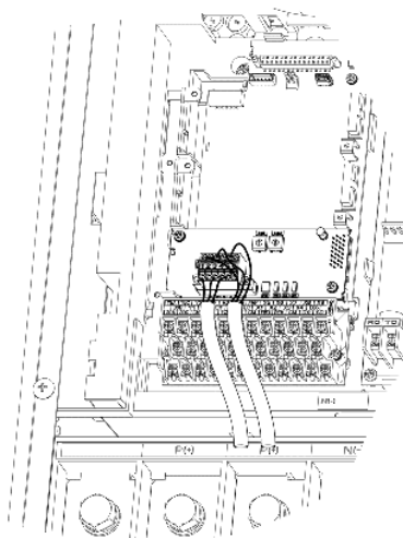
FRENIC-HVAC 90kW の例
