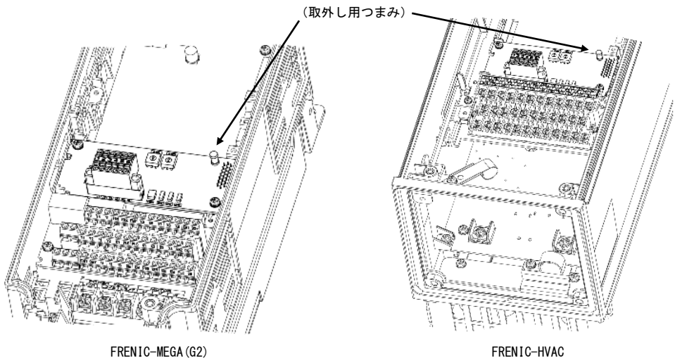
図 3.3 取付け完了 (A-port 取付け時)
