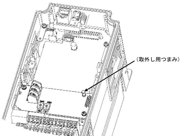
図 3.3 取付け完了
